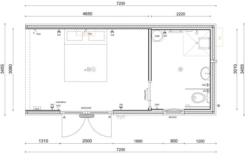
Begane grond 1:15
