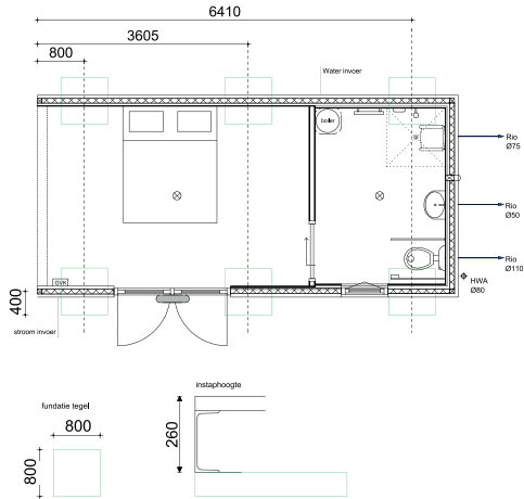
Fundatie tekening 1:25
