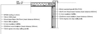
Dak opbouw 1:10
